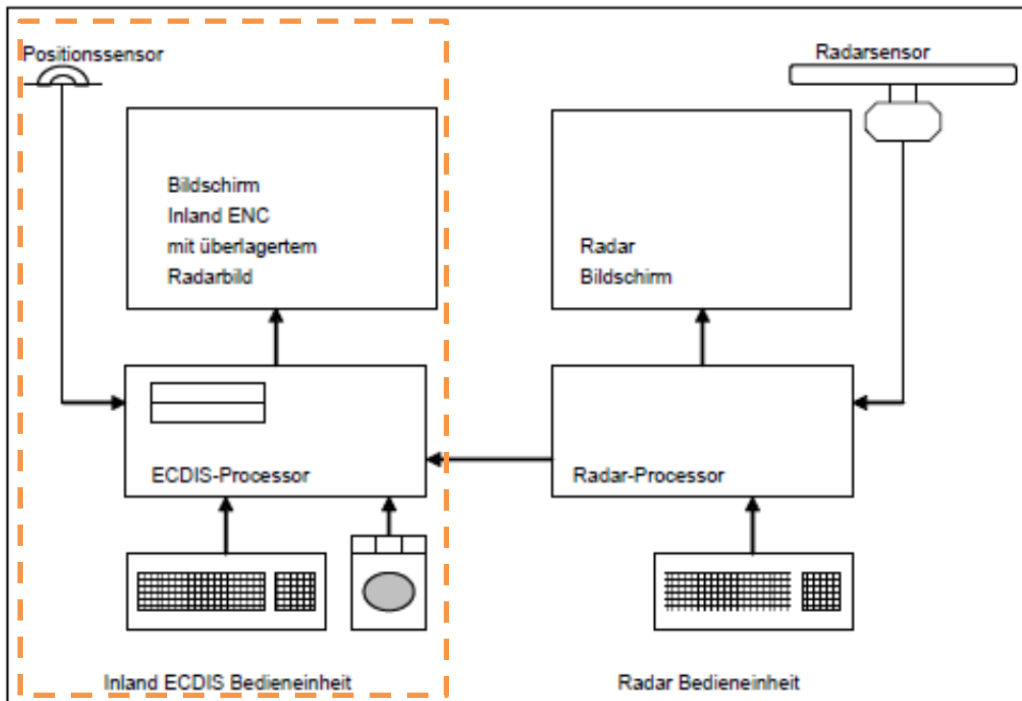
Anhang Bild 1: Inland ECDIS Gerät, autarkes Gerät mit Verbindung zur Radaranlage (Systemkonfiguration 2)
